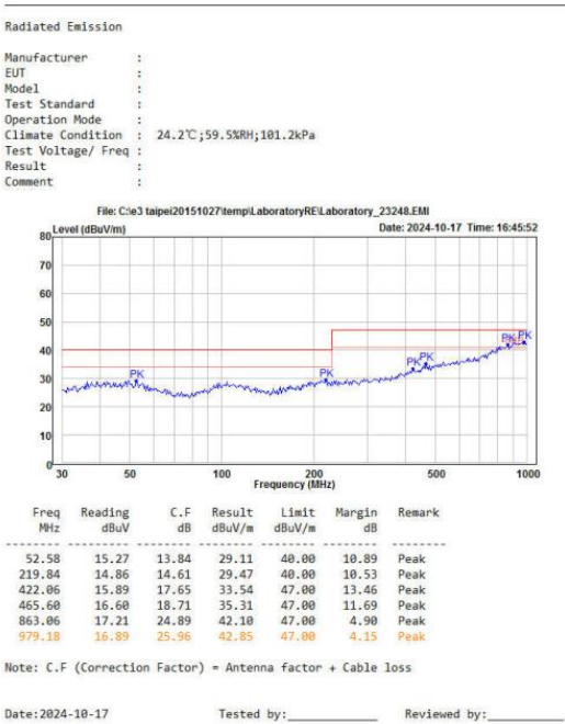
图 6-6 辐射测试水平方向
