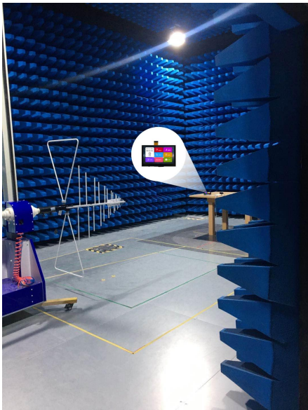
图 6-5 辐射测试图
